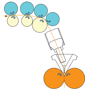
ÇIKIŞ HUNİSİ
